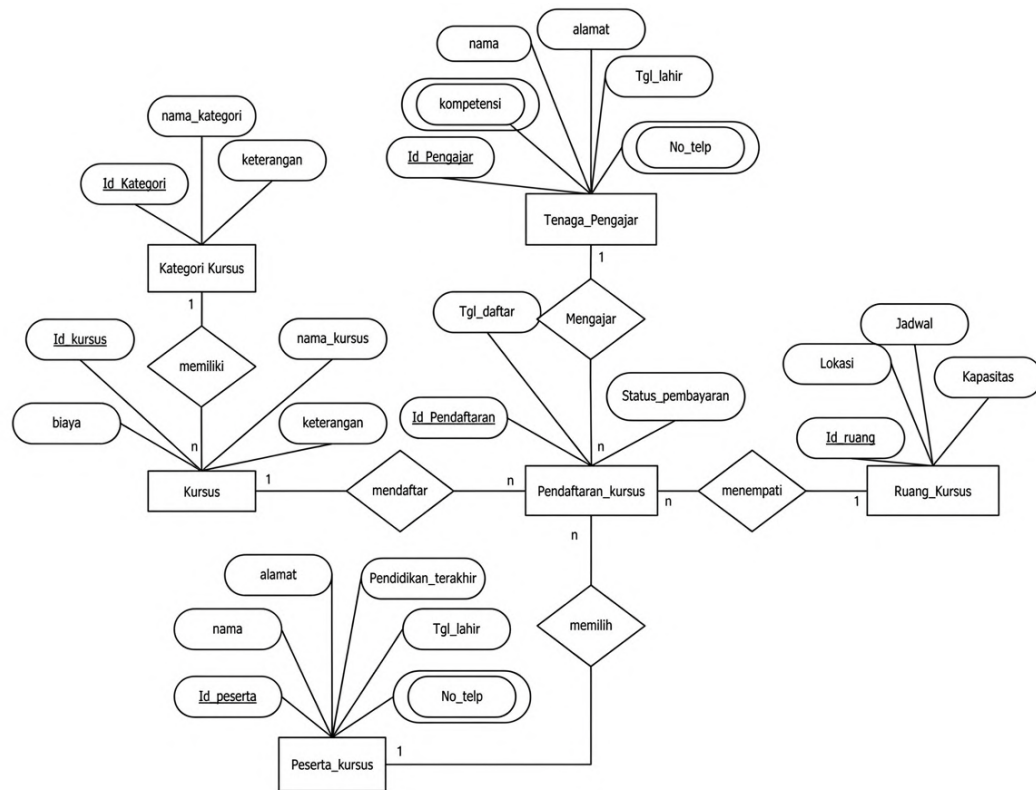
Gambar 1 Gambar ERD/ Diagram ER
